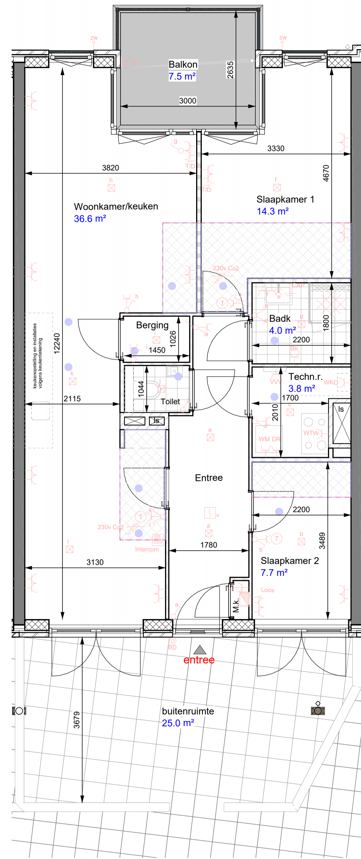
Plattegrond
